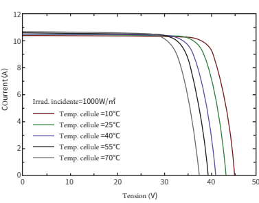
Courbe I-V à différentes irradiances (SPP280NHEH)
